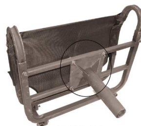
BILD 18 Installation der oberen Sitzstütze
